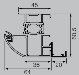
Eenzijdige verbreding
